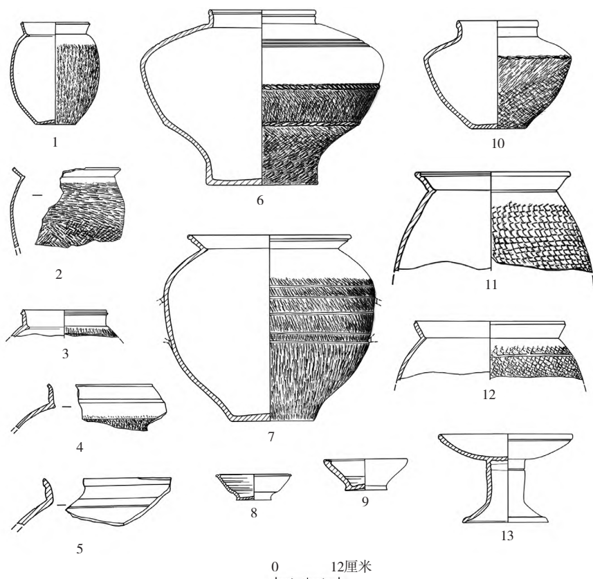
图一三 第二期陶器
