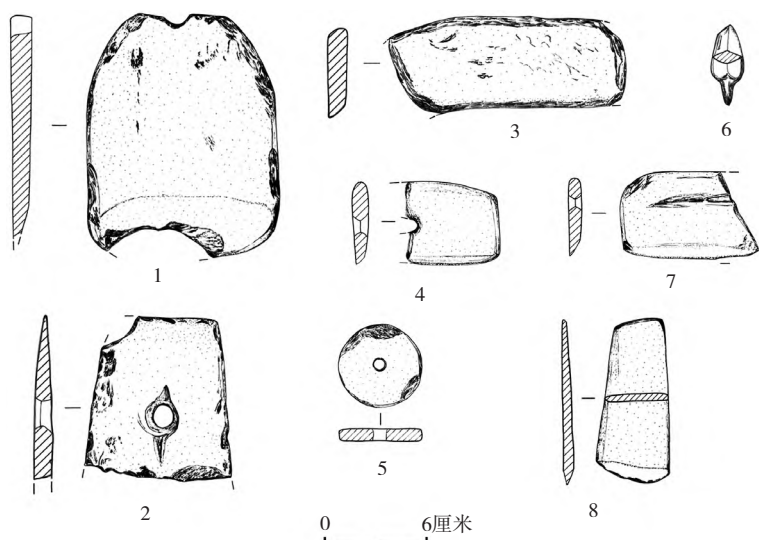
图一六 第二期石器
