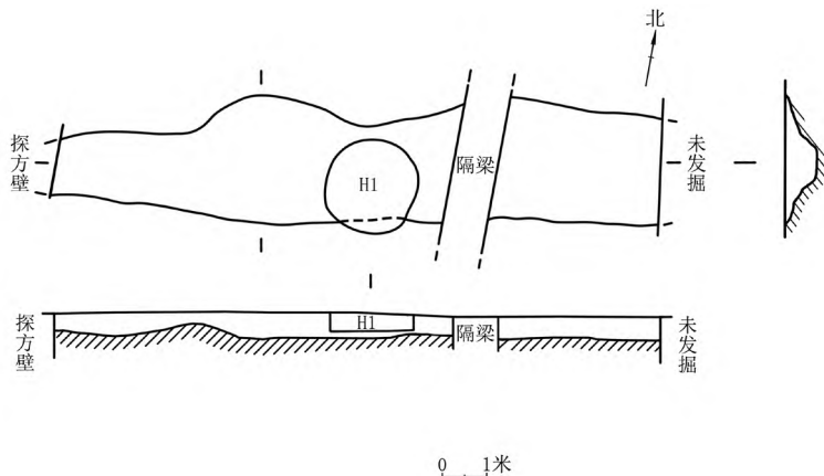
图五 G1平、剖图
