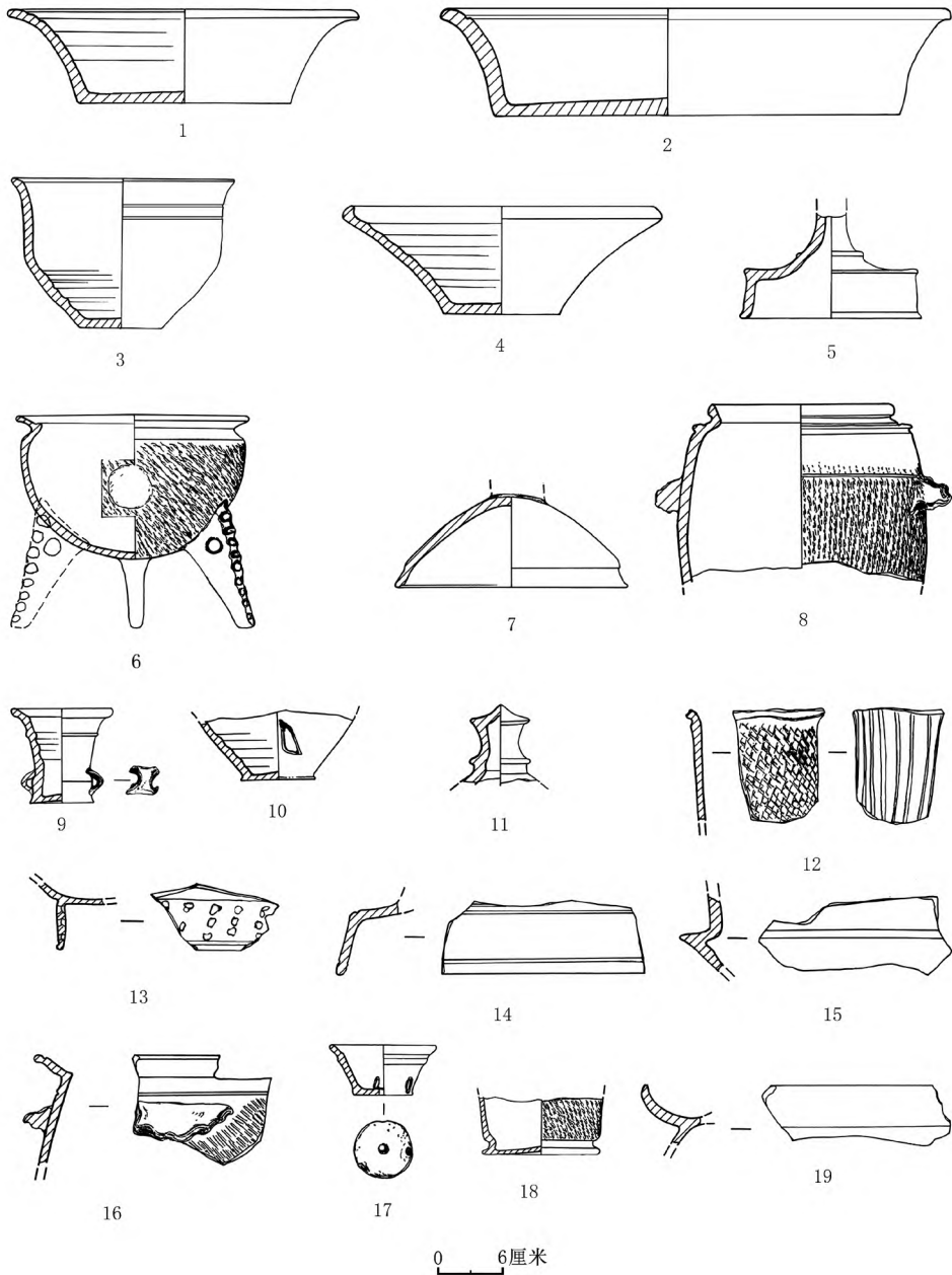
图一四 第二期陶器
