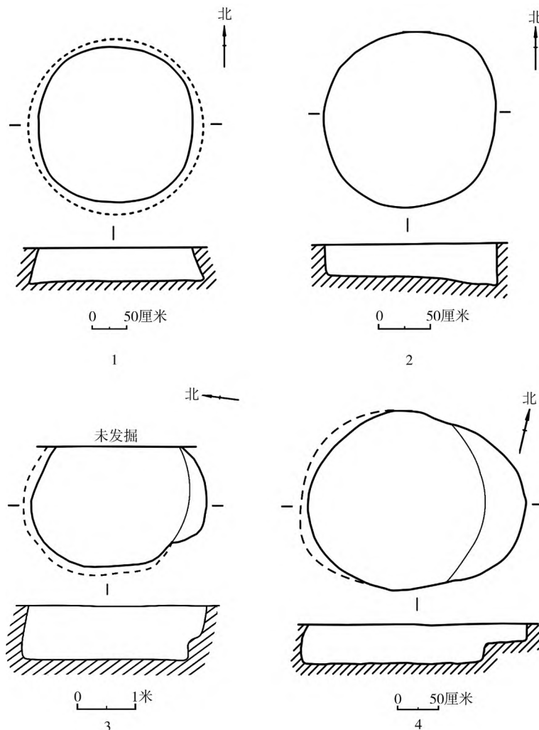
图六 第二期遗迹平、剖图（一） 1. H22 2. H30 3. H31 4. H9
