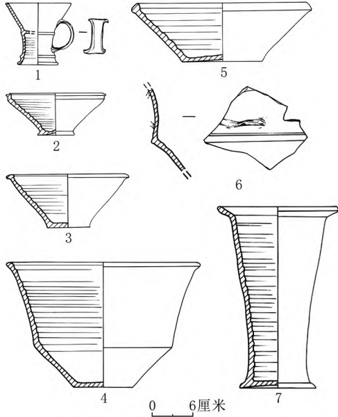
图一 第一期陶器
