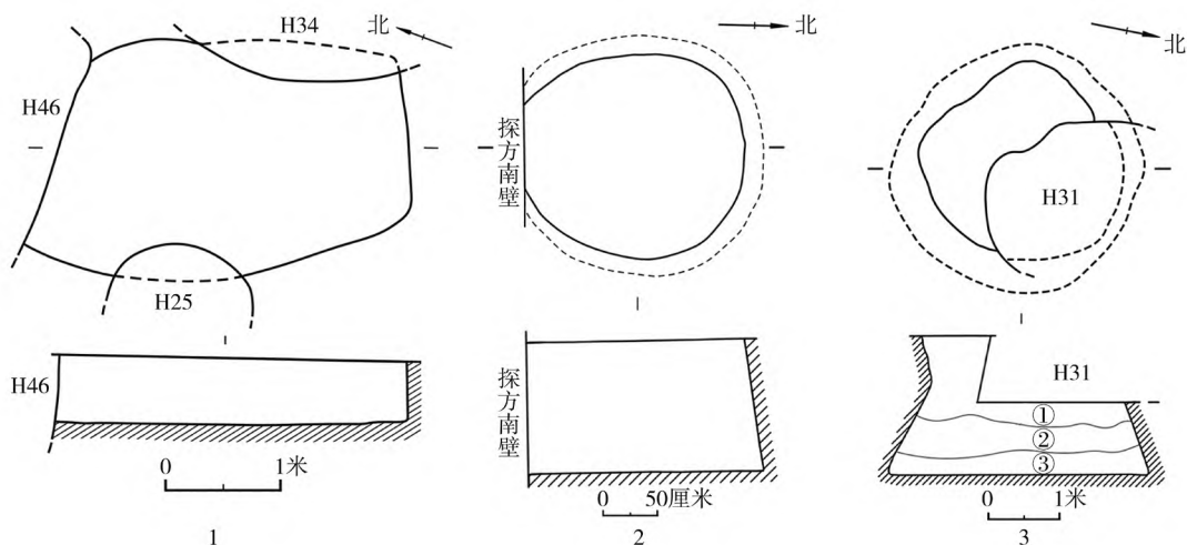
图四 第一期遗迹平、剖图 1. H47 2. H8 3. H42
