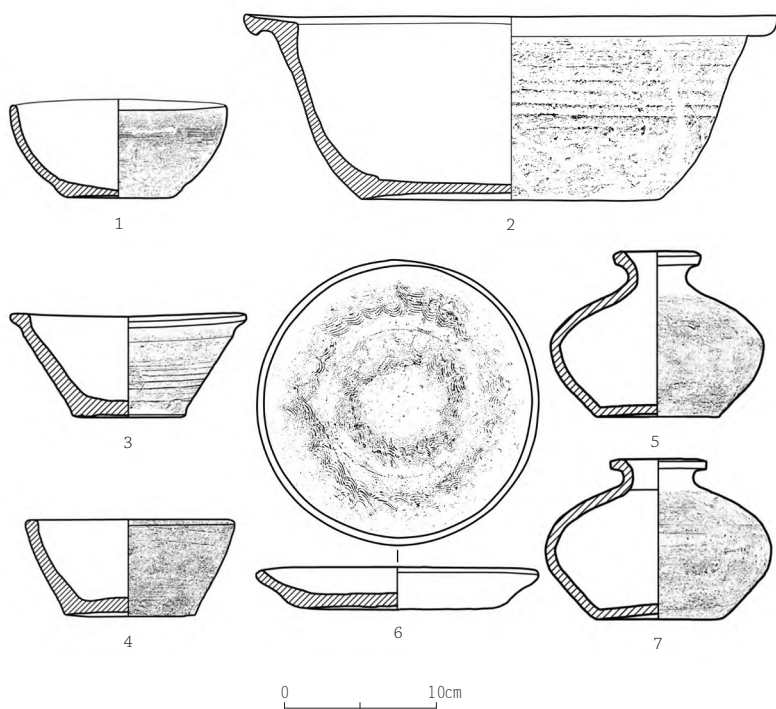
〔图十六〕出土陶碗、盆、壶、盘
