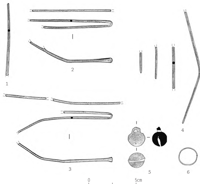
〔图二十〕出土铜器
