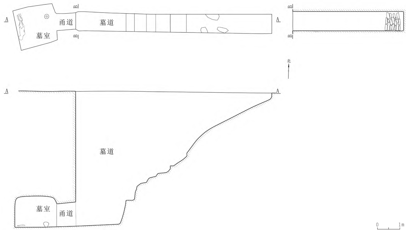
〔图六〕M34平面图
