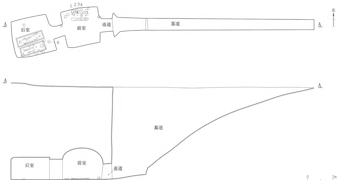
〔图十四〕M44平面图
