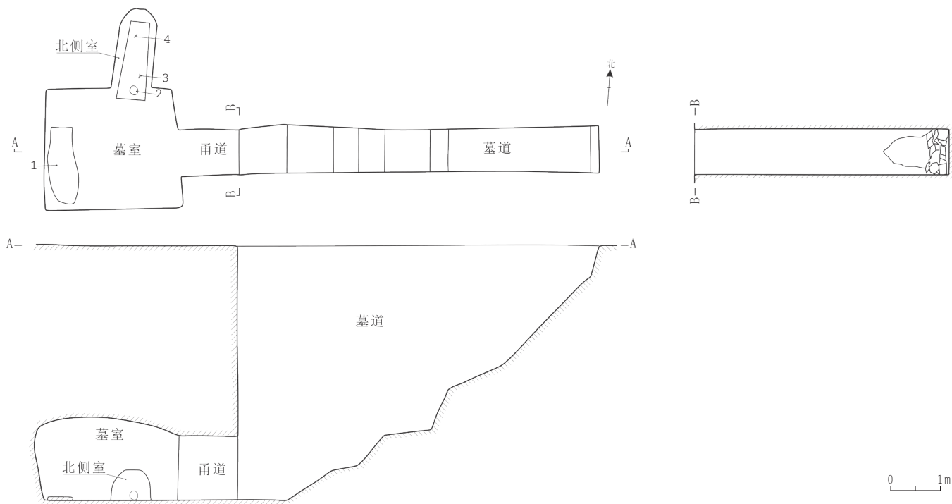
〔图十二〕M32平面图
