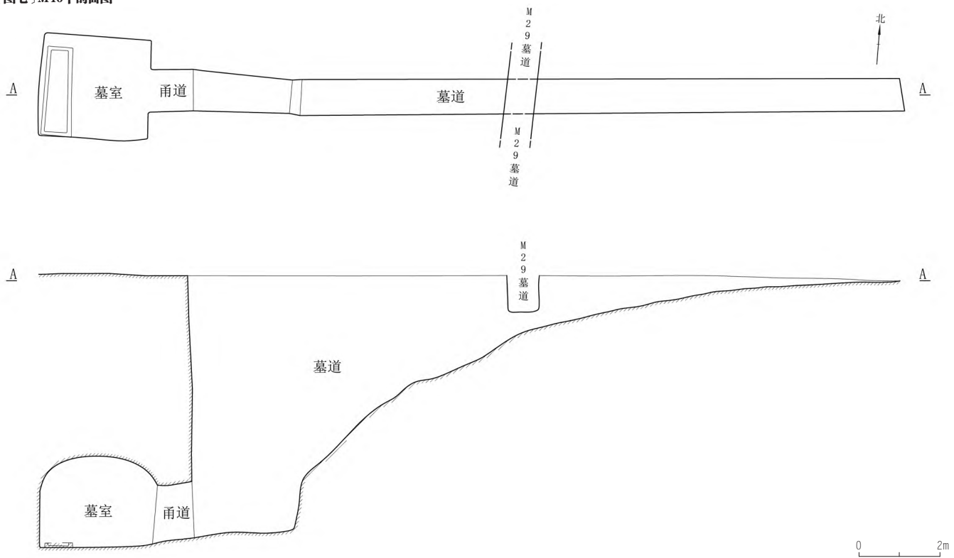
〔图七〕M40平面图
