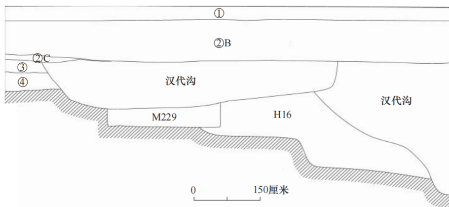
图三 T6 南壁剖面图
