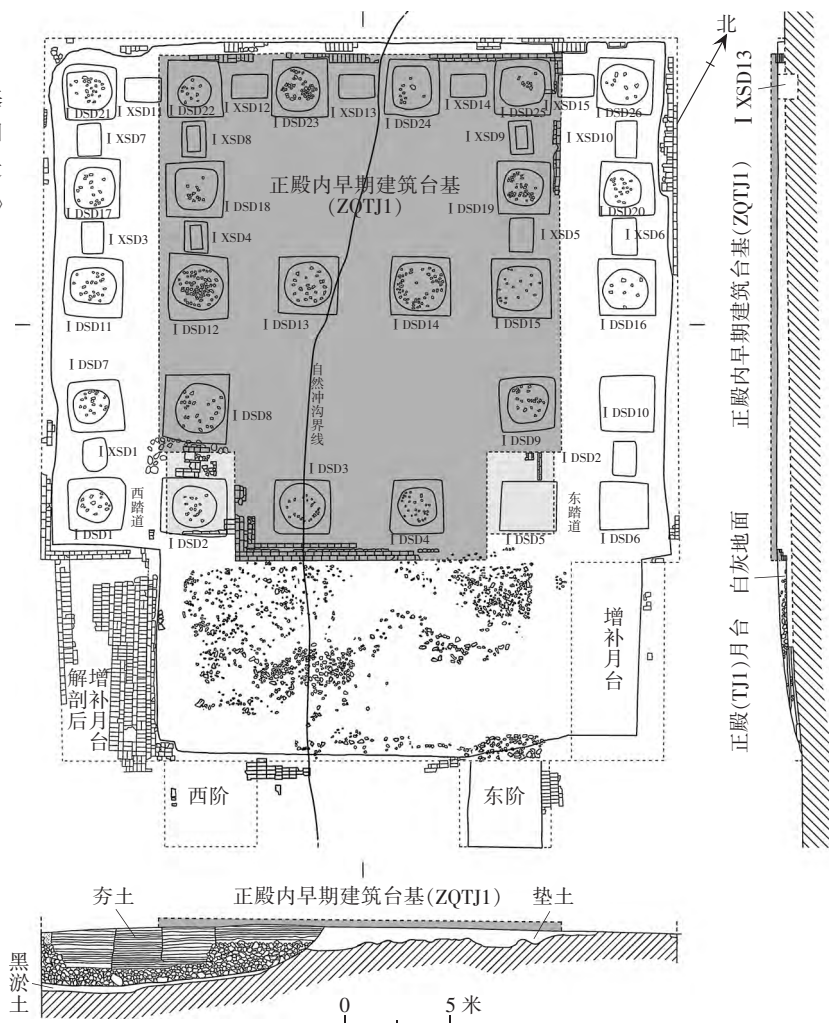
图六 新立建筑基址早期台基(ZQTJ1)及晚期台基(TJ1)平、剖面图(据《辽宁北镇新立辽代遗址一号基址 2018 年发掘简报》图六改绘)
