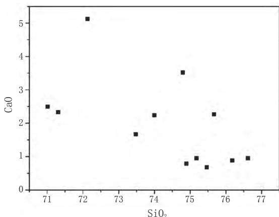
图三 阿敦乔鲁釉砂 \text{SiO}_2 、CaO 散点图
