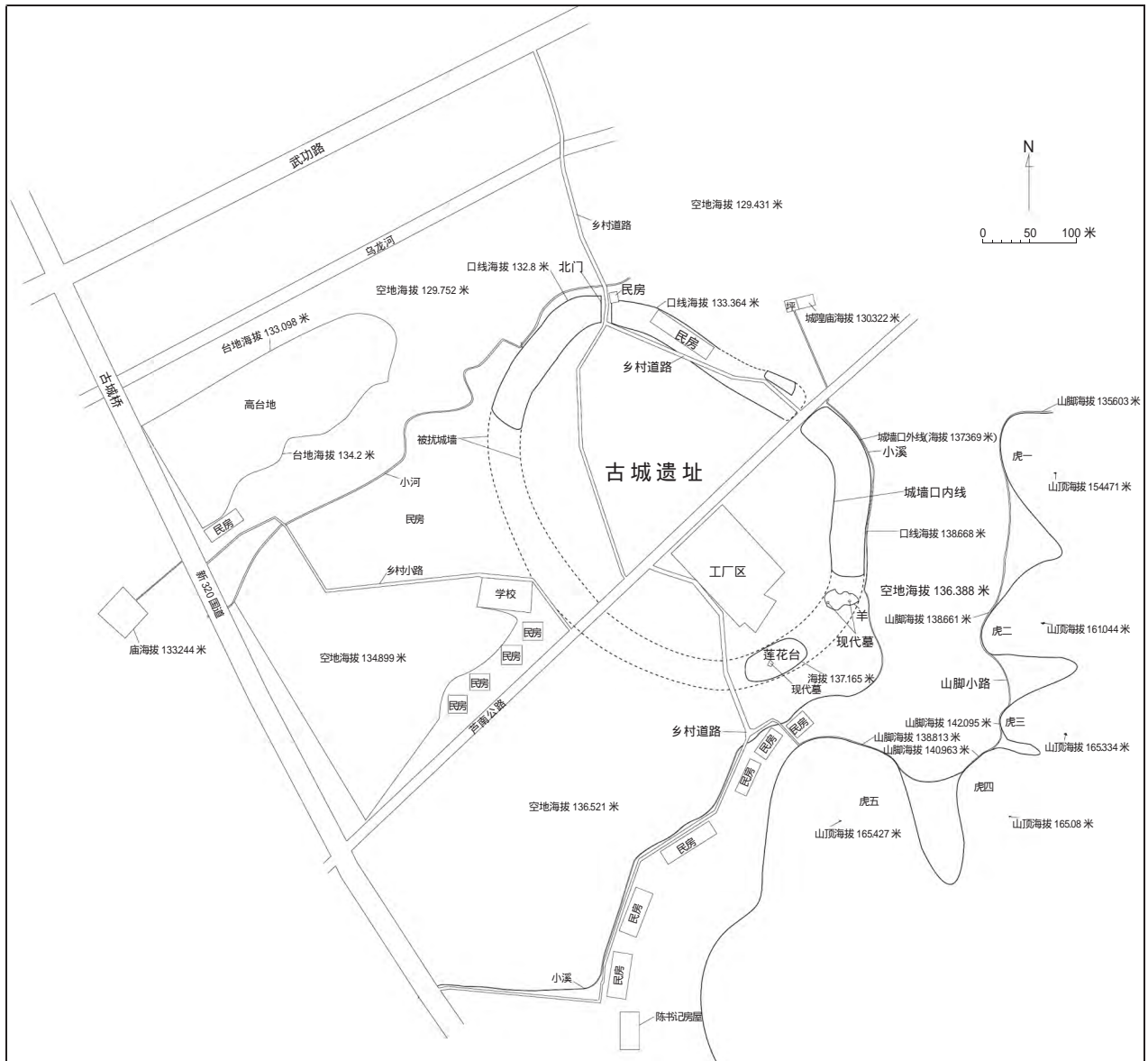
图三 芦溪古城平面测绘图(城墙北段、东城地表犹存,西现段据钻探绘制)
