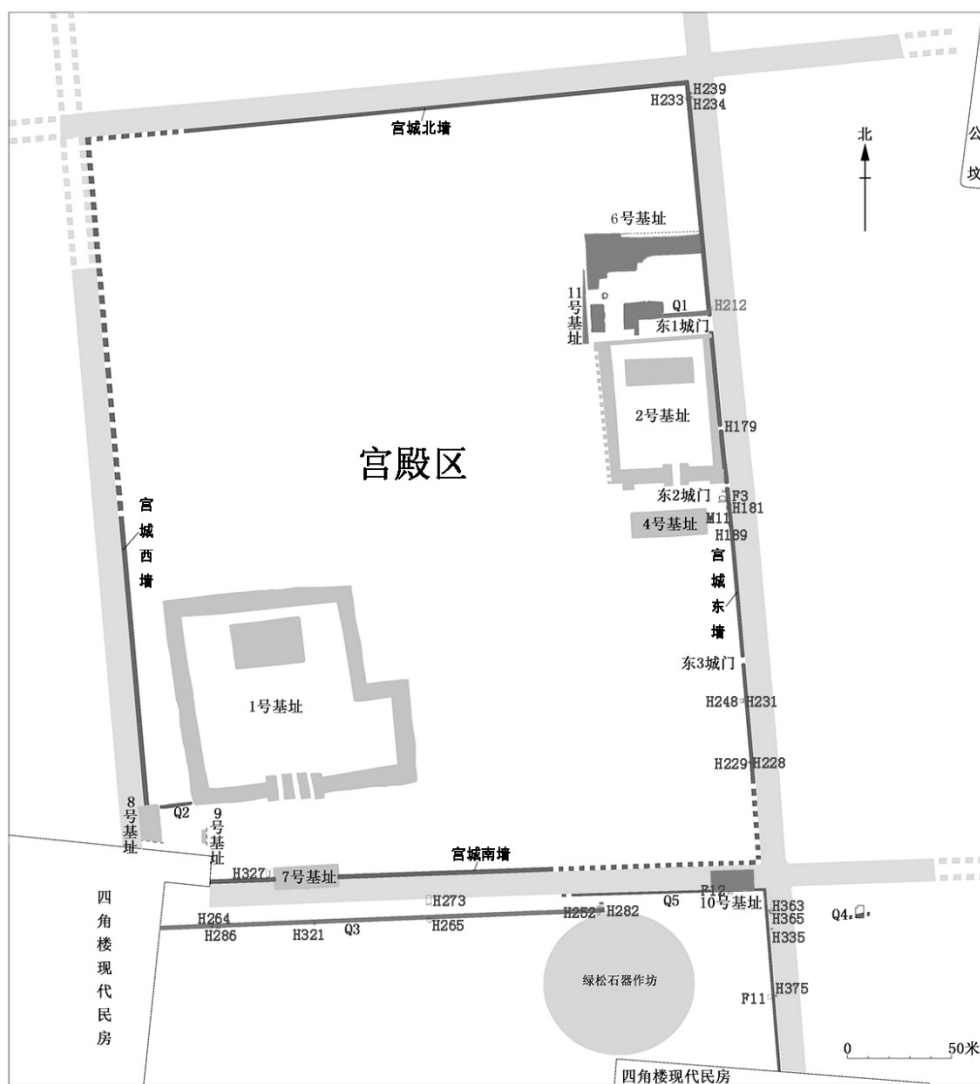
图一 中心区道路网络、宫城城墙及相关遗迹平面图
