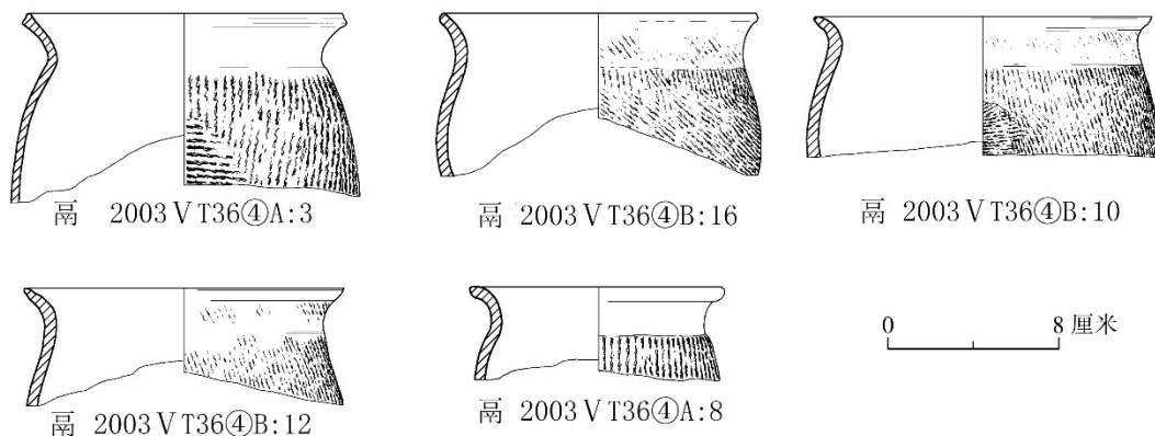
图六 2003 VT36④层出土陶鬲
