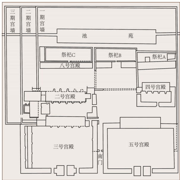
图四 偃师商城5段宫城平面布局示意图
