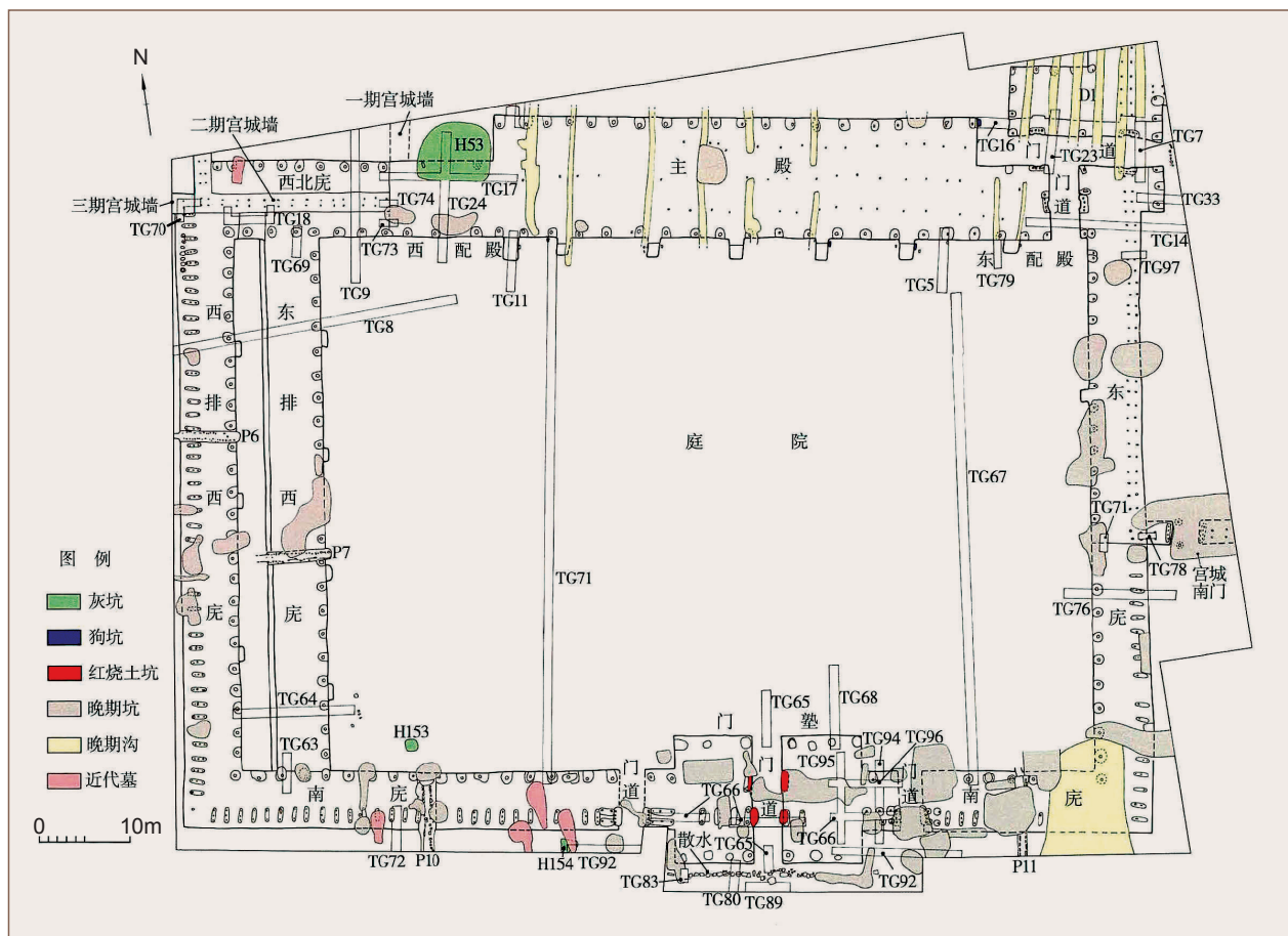
图一 三号宫殿建筑基址平面图
