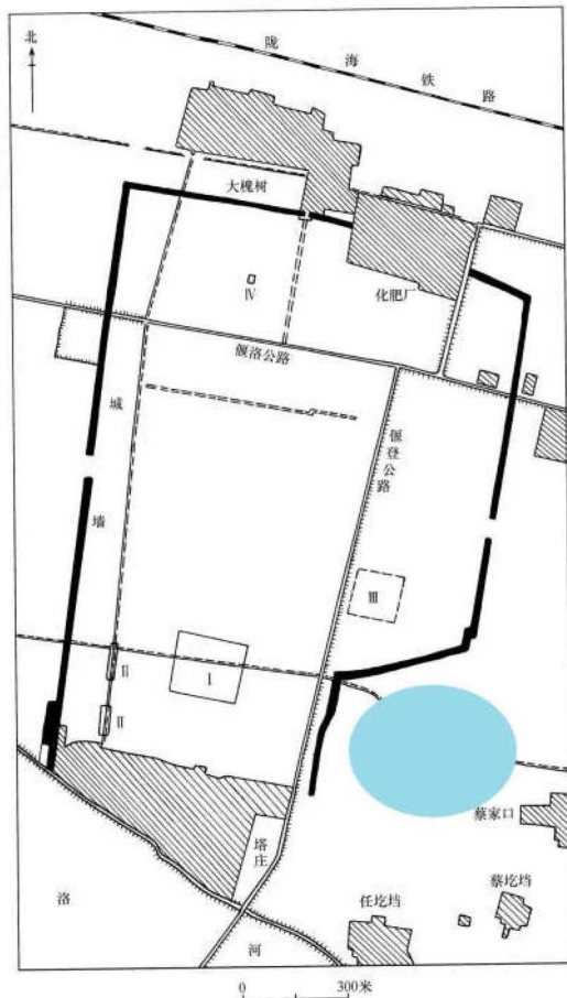
图二 1983年偃师商城勘探遗迹图
