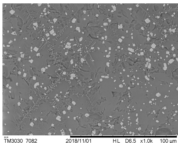
图五 450113 样品背散射电子像 方形锡石颗粒及枝状氧化亚铜晶体 弥散分布于铅硅酸盐基体之上
