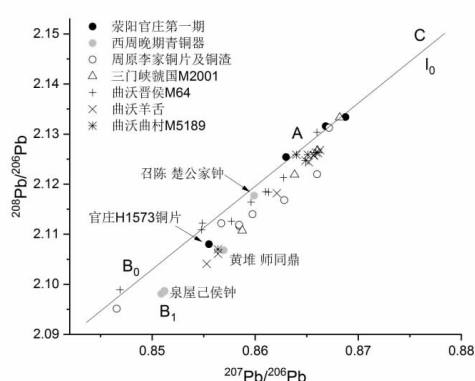
图一〇 西周晚期至春秋初年中原地区部分青铜器及铸铜遗物的铅同位素比值
