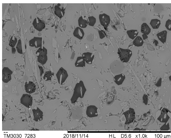
图六 450108 样品背散射电子像 方形及条状锡石颗粒(浅灰色) 与胞状锡铁硅酸盐相(黑灰色)
