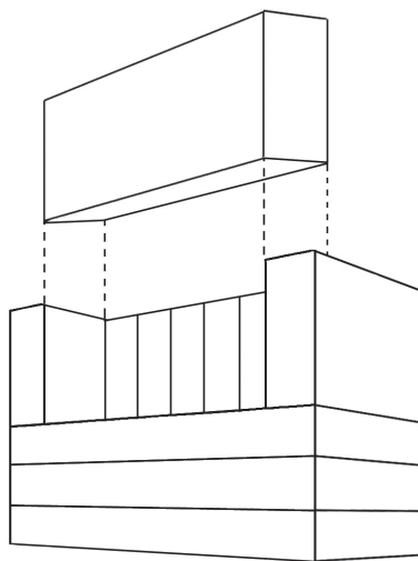
图一 髹砖层夹砌陡板示意图
