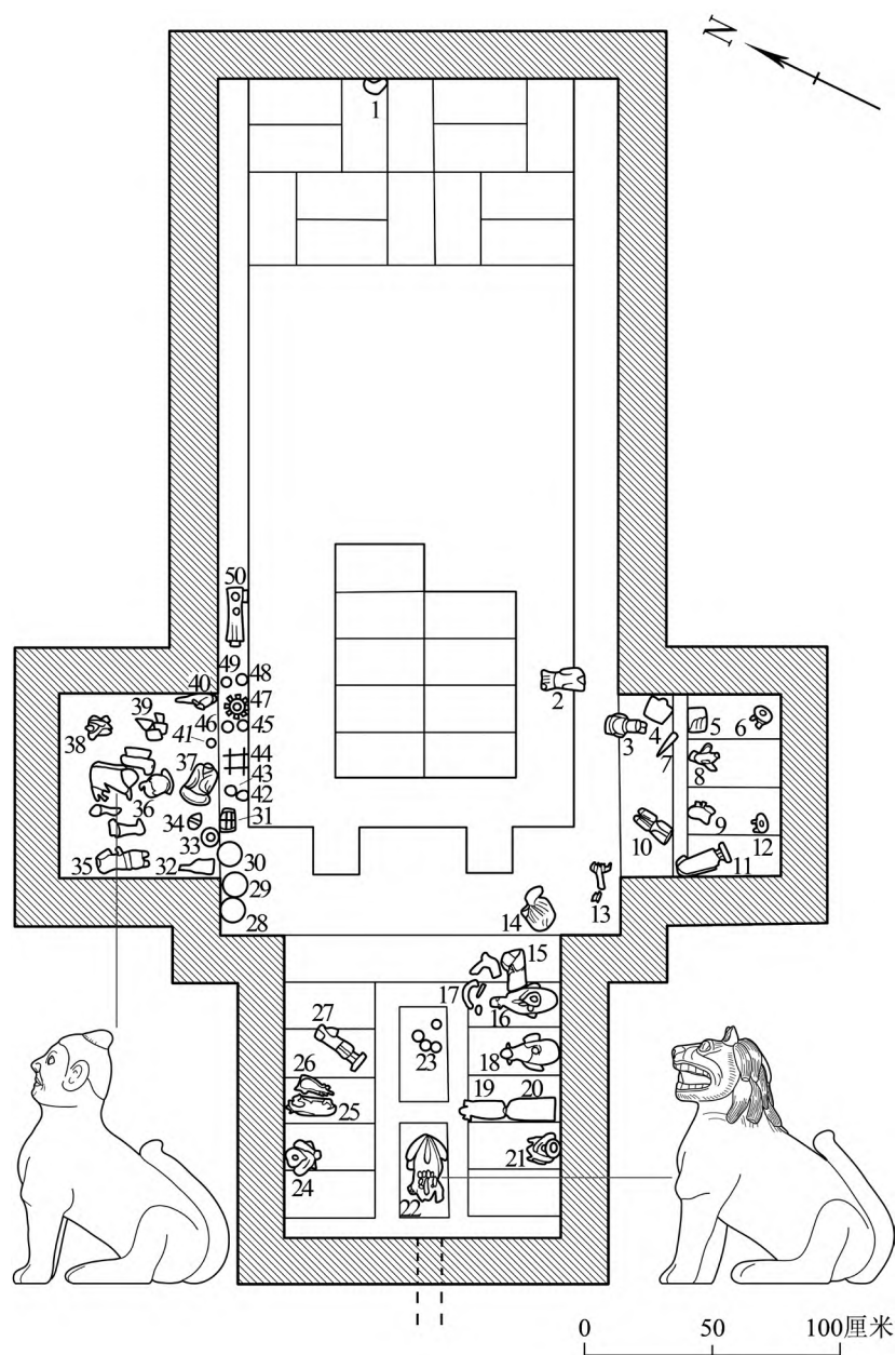
图四 武昌何家垅M439平面图及镇墓兽出土位置 (改绘自《武昌隋唐墓》)
